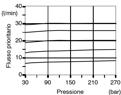
Diagramma Portata-Pressione
