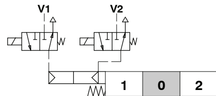
Simbolo dettagliato
