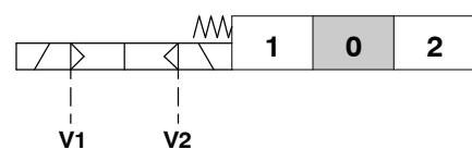
Simbolo semplificato
